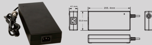
Appearance Size / 外观尺寸
